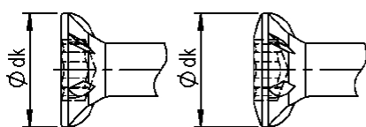
Kleiner (Linsensenk-) Kopf
