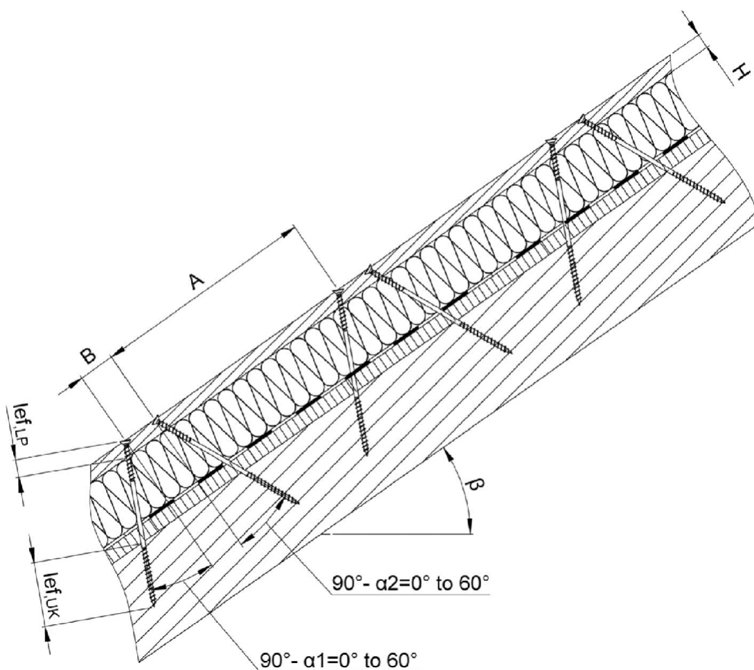
Obrázek A.4.4 Upevnění střešní izolace ke krokvím - principiální obrázek se šrouby rozmístěnými pod různým sklonem
