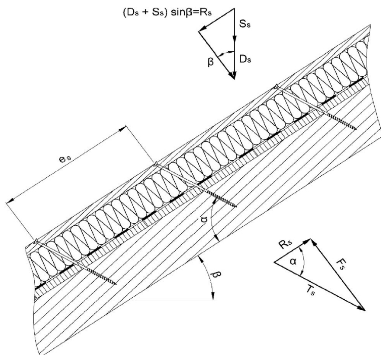
Obrázek A.4.3 Jednotlivá zatížení F_s kolmo na kontralatě, působení zatížení v oblasti hlavy šroubu
