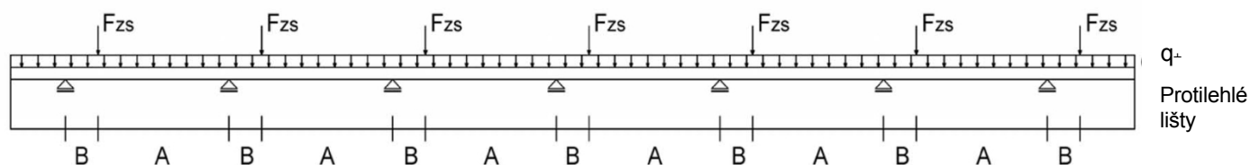
Obrázek A.4.5 Průběžná kontralátě vystavená stálému liniovému zatížení na povrchu střechy q_{\perp} a soustředěnému zatížení od předeprtých šroubů F_{zs}
