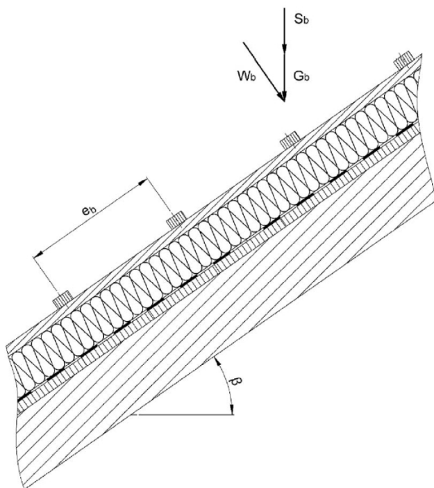
Obrázek A.4.2 Jednotlivá zatížení F_b v pravém úhlu k protilehlým latím
