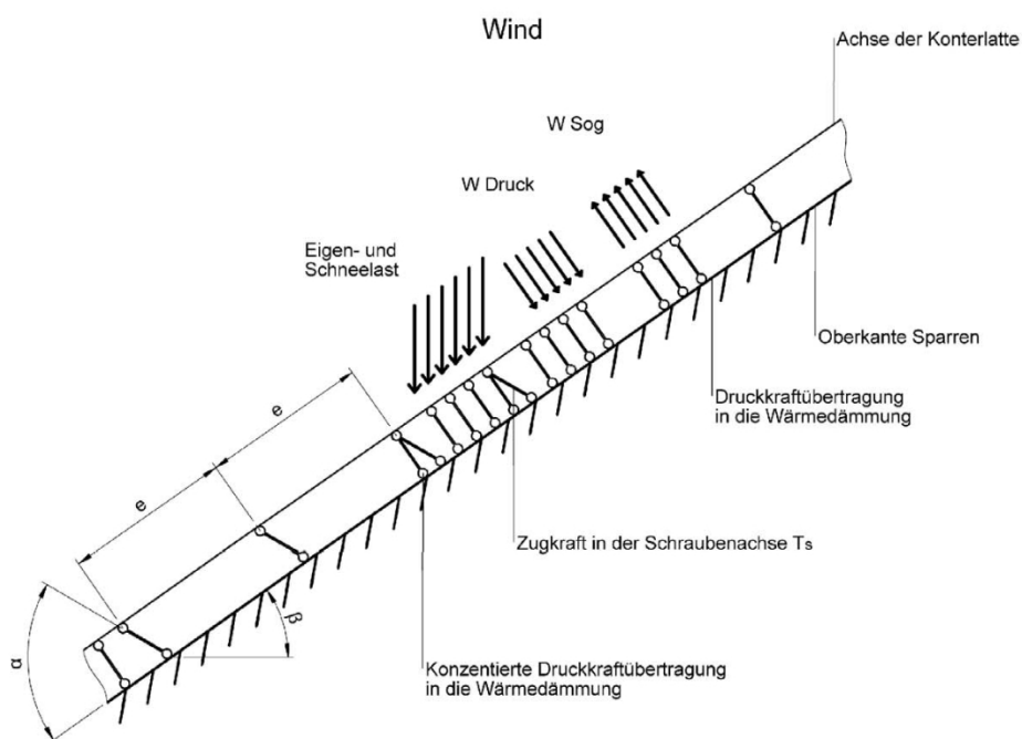
Obrázek A.4.1 Upevnění střešních izolačních systémů ke krokvím - konstrukční model pro paralelní šrouby
